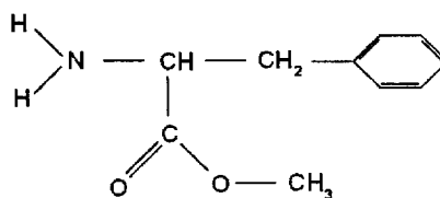
ester méthylique de la phénylalanine
