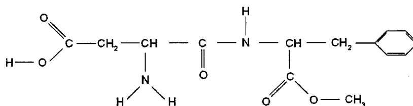
molécule d'aspartame
